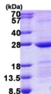
15% SDS-PAGE (3µg)
